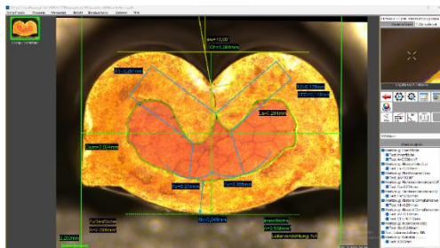
Fertig vermessenes Schliffbild mit X-Scan
